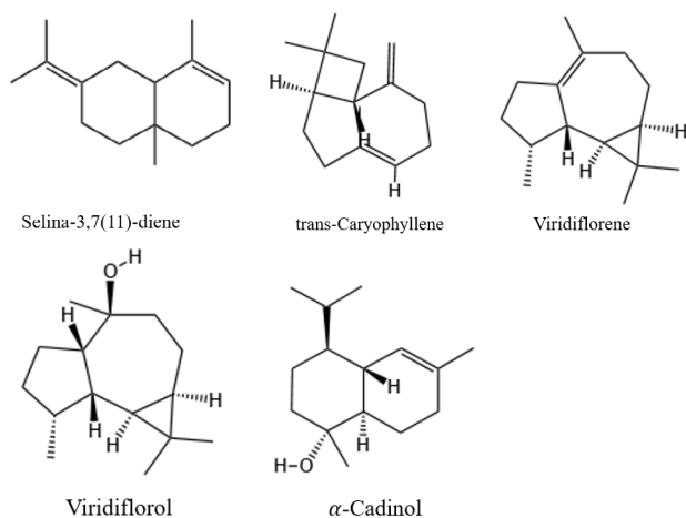
Figura 2. Estrutura moleculares 2D dos ligantes com melhor afinidade de ligação com PfENR.
