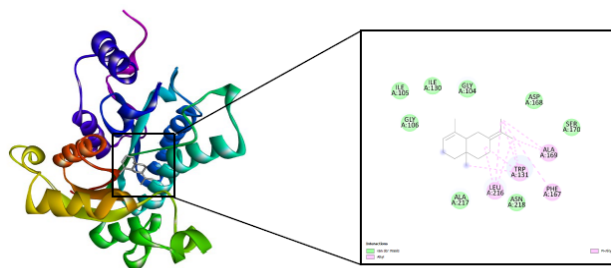
Figura 3. Selina-3,7(11)-diene acoplado a PfENR.
