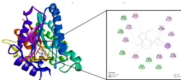
Figura 4. Viridifloreno acoplado a PfENR
