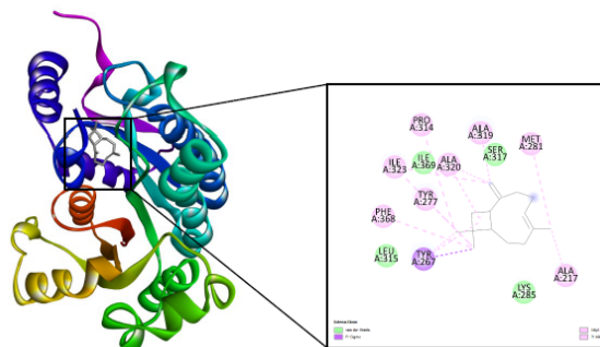
Figura 6. trans-Cariofileno acoplado ao PfENR
