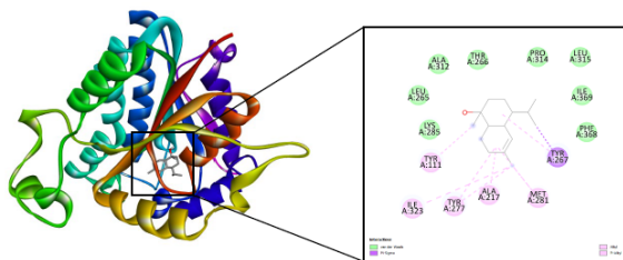
Figura 5. \alpha -Cadinol acoplado ao PfENR.
