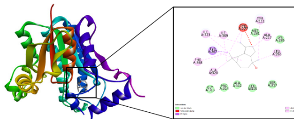
Figura 7. Viridiflorol acoplado ao PfENR
