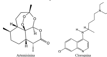
Figura 8. Estruturas moleculares 2D de antimaláricos comercializados
